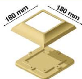
Πέλμα κολώνας 1500
